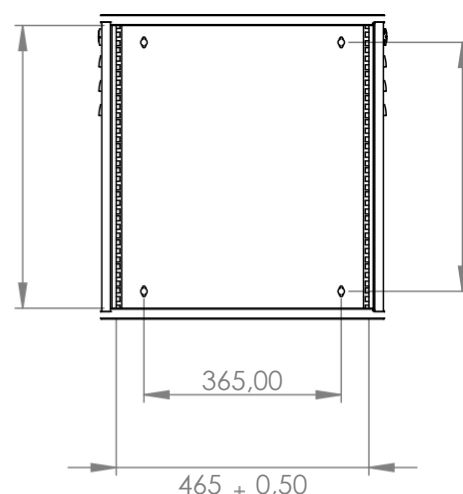
465 ± 0,50 Entre Centros Vista Frontal Sem Porta
