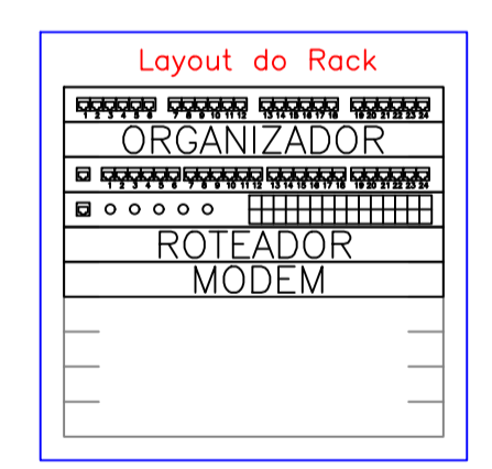
LAYOUT DO RACK SEM ESCALA
