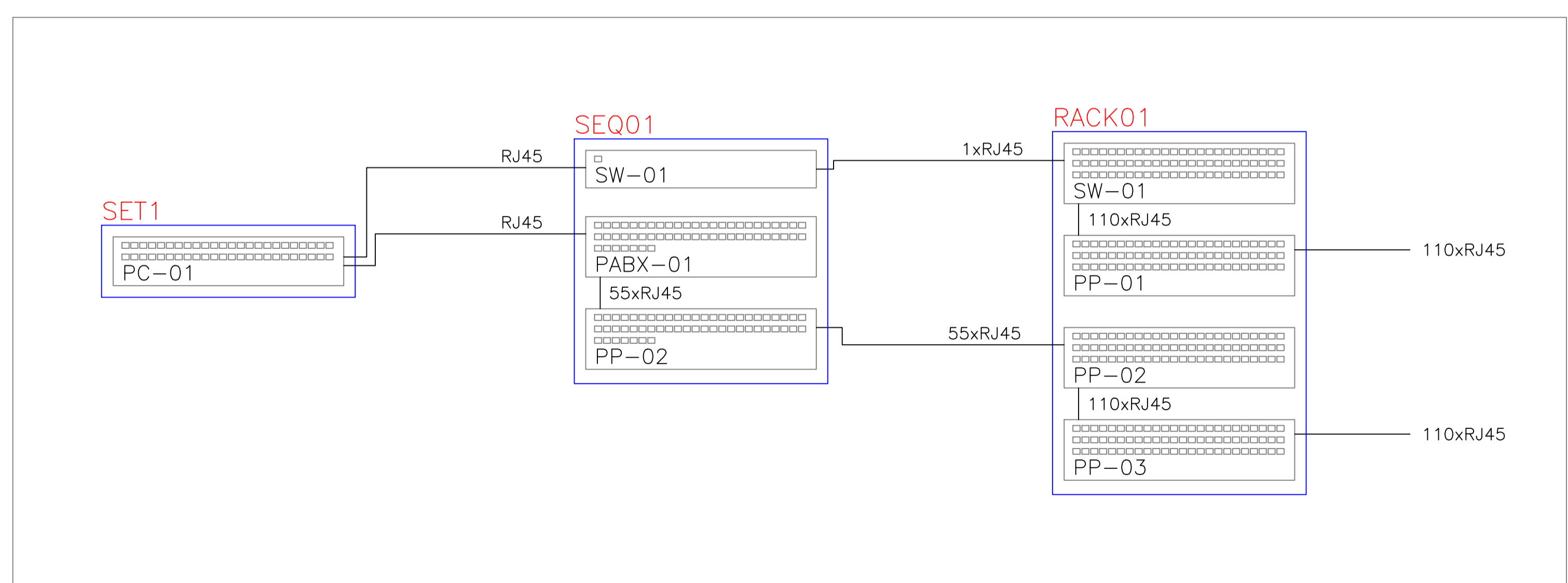
DIAGRAMA DE CABEAMENTO SEM ESCALA
