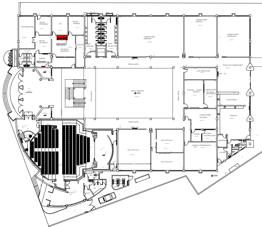
PLANTA - PISO TÉRREO - UNIDADE II ESCALA 1:100
