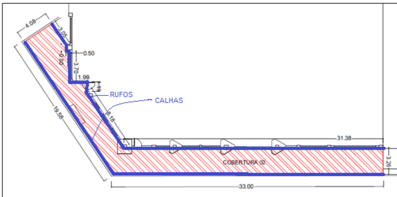
Figura 2: Dimensões da cobertura 02 (sem escala)
