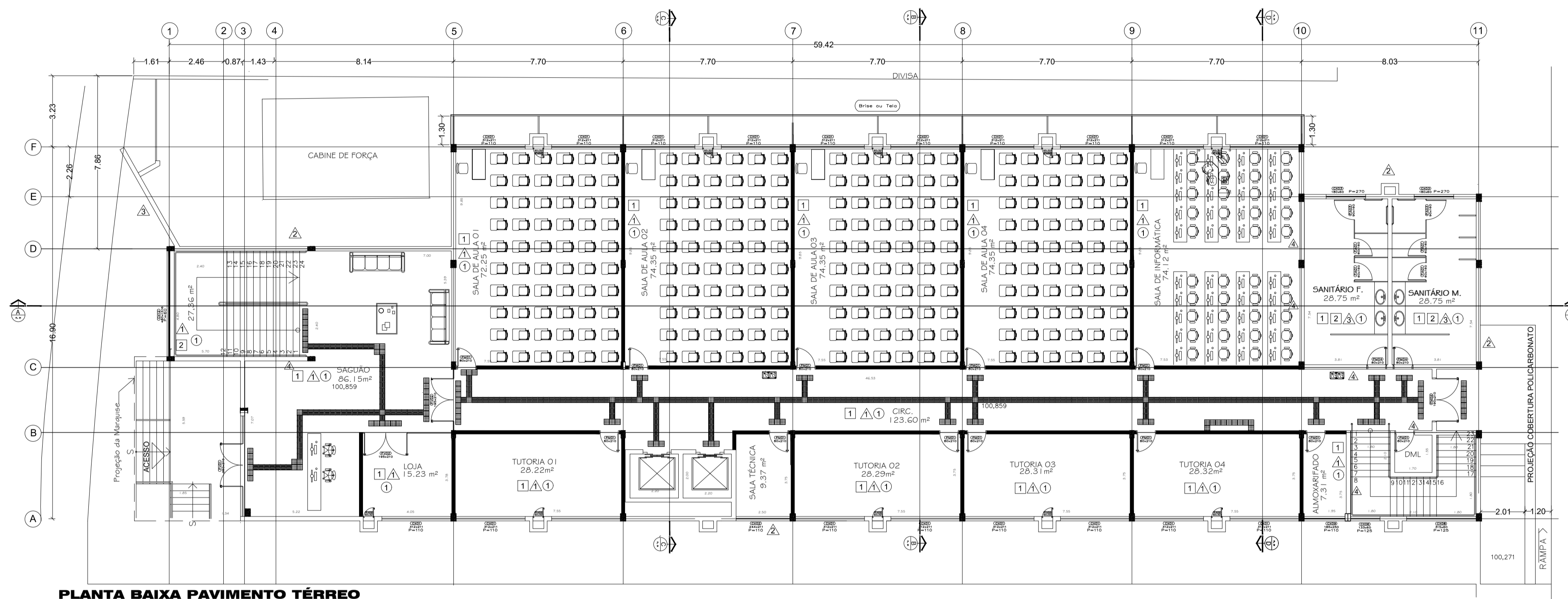
PLANTA BAIXA PAVIMENTO TÉRREO ESCALA 1:100
