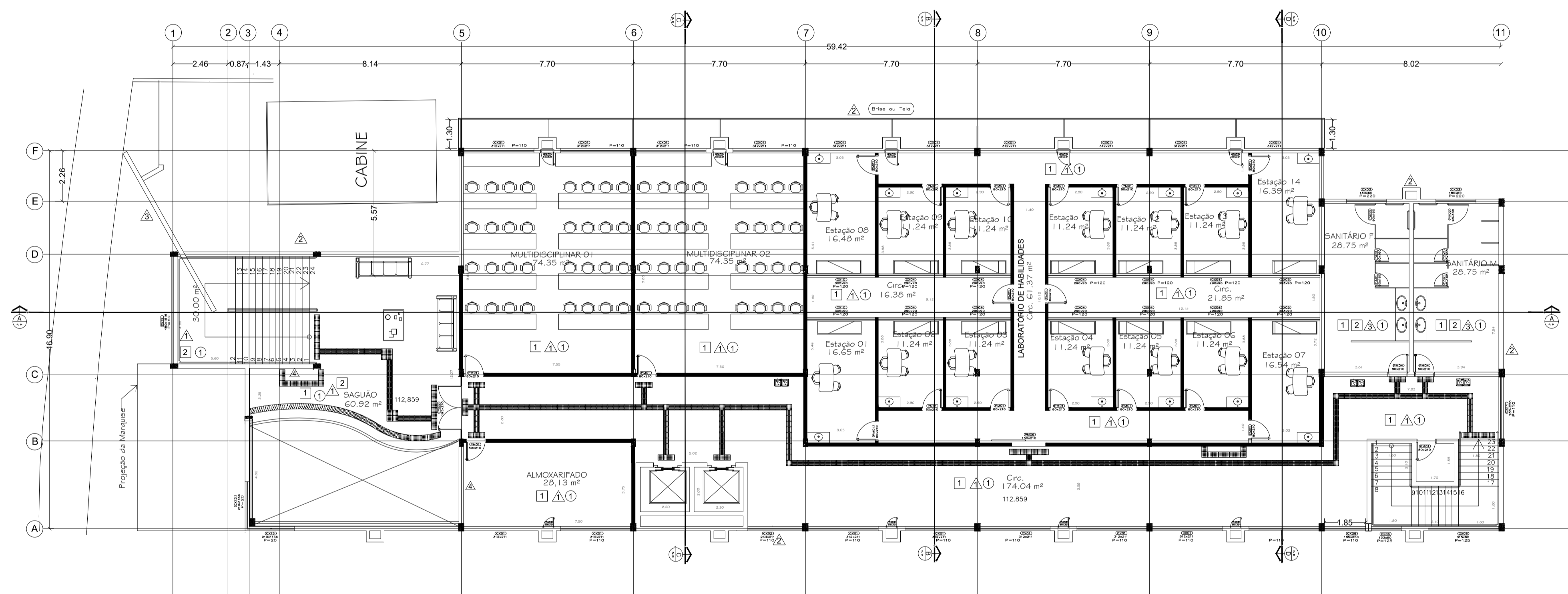
PLANTA BAIXA 3º PAVIMENTO ESCALA 1:100
