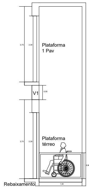
CORTE A
