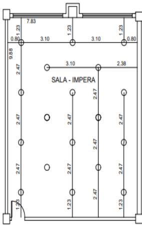
LOCAÇÃO LUMINÁRIAS ESCALA 1:100
